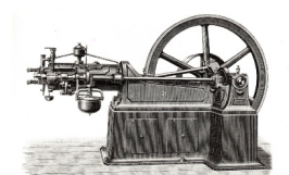
1876 Otto-Viertakt-Gasmotor
